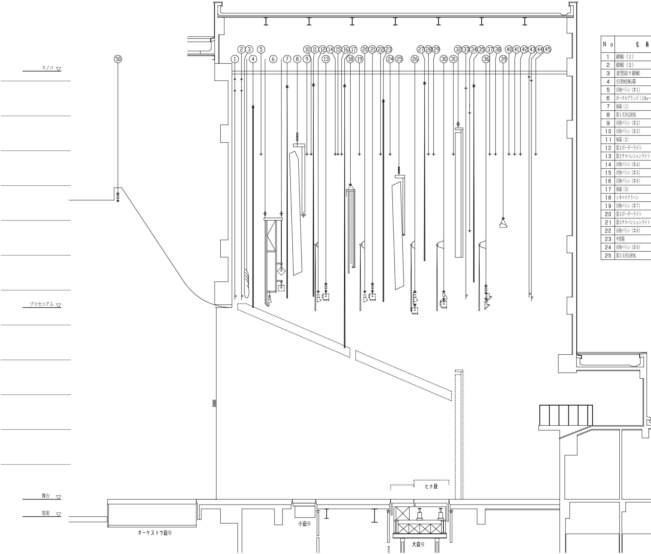
尼崎市総合文化センター 大ホール 舞台吊物断面図 S=1/100
